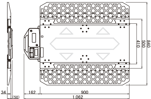
パッド外観図
