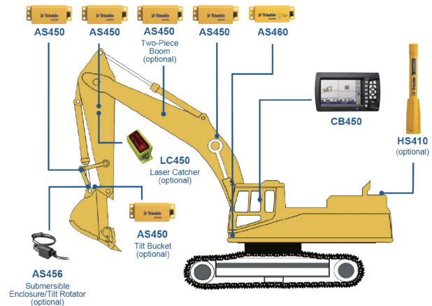
GCS900 2D for Excavators システム構成図
