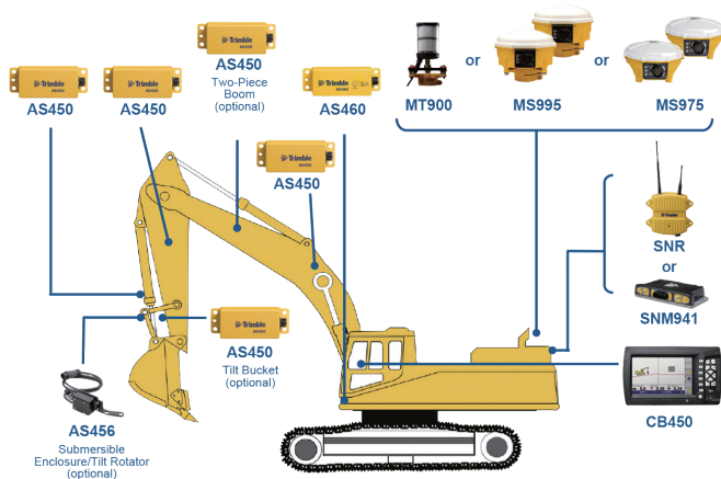
GCS900 3D for Excavators システム構成図
